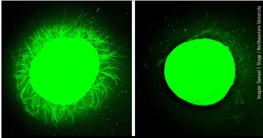
Crecimiento de neuritas de un organoide de médula espinal humana tratado con “moléculas danzantes” de movimiento rápido (izq.) comparado con uno tratado con moléculas de movimiento lento (der.) utilizando sustancias químicas similares.
